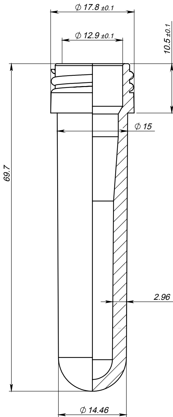
SECTION B-B SCALE 2 : 1
