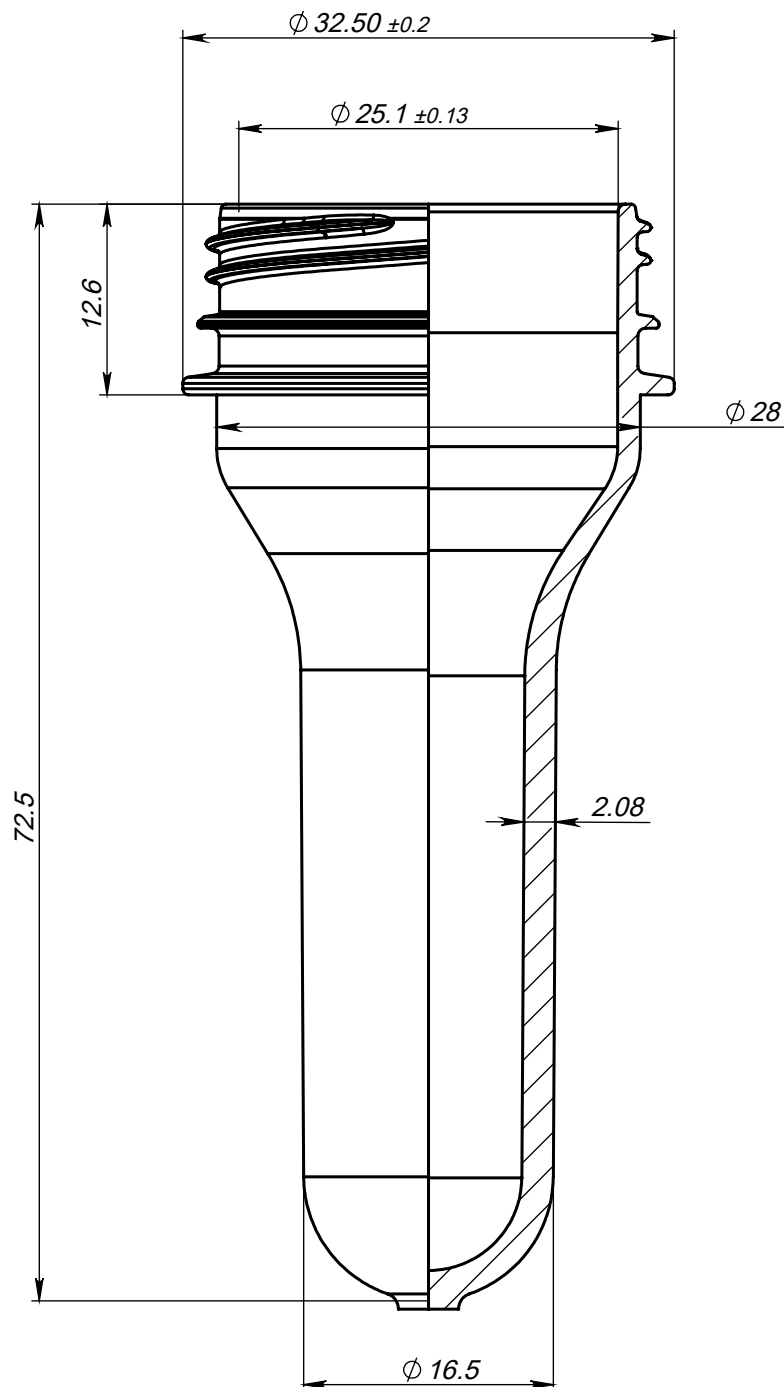
SECTION B-B SCALE 2 : 1
